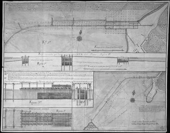
Fig. 2. Antonio de Arévalo. Plano y perfiles del Malecon que se está construyendo de orden de S. M. desde el día 11 de Noviembre de 1771 para cerrar la abertura de Boca-grande, entrada á la Bahía de Cartagena de Yndias, 1774.
